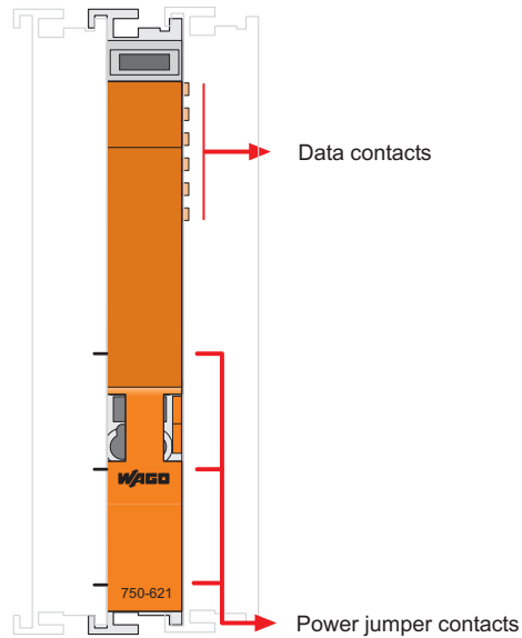
Fig. 2.1.1-1: Separation Module 750-621
